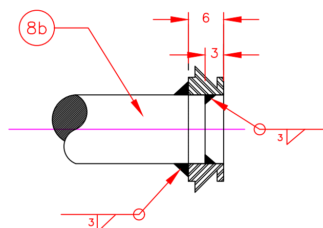
DETALLE 2
