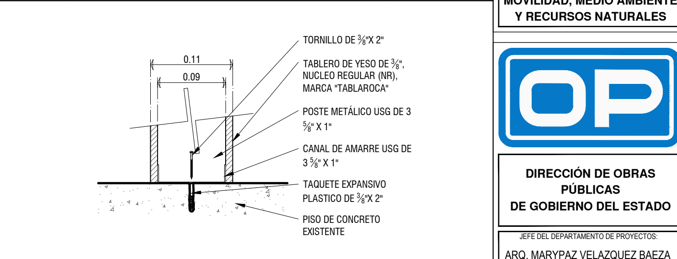
DB09 DETALLE DE ANCLAJE EN PISO DE MURO DE TABLAROCA ESC: 1 : 5
