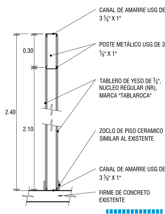
DA06 DETALLE DE MURO DE TABLAROCA ESC: 1:20
