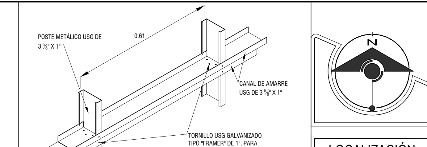
DB06 DETALLE DE TRASLAPE DE POSTES EN MURO DE TABLAROCA ESCHEMA
