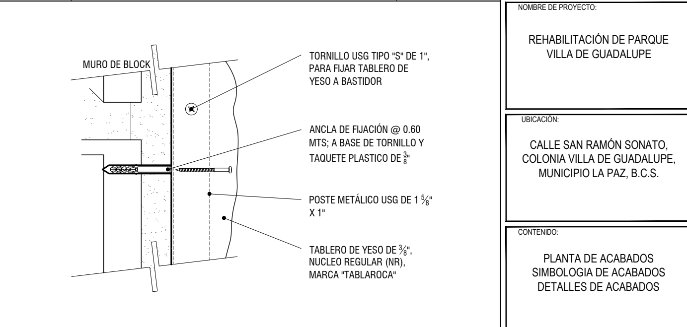
DB10 DETALLE DE ANCLAJE EN MURO DE MURO DE TABLAROCA ESCHEMA
