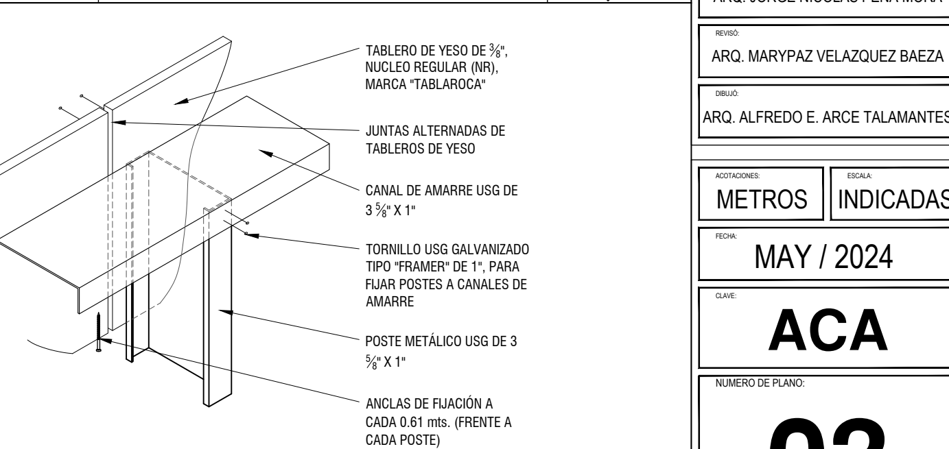
DB11 DETALLE DE AMARRE SUPERIOR DE PERFILES DE MURO DE TABLAROCA ESC: 1 : 5
