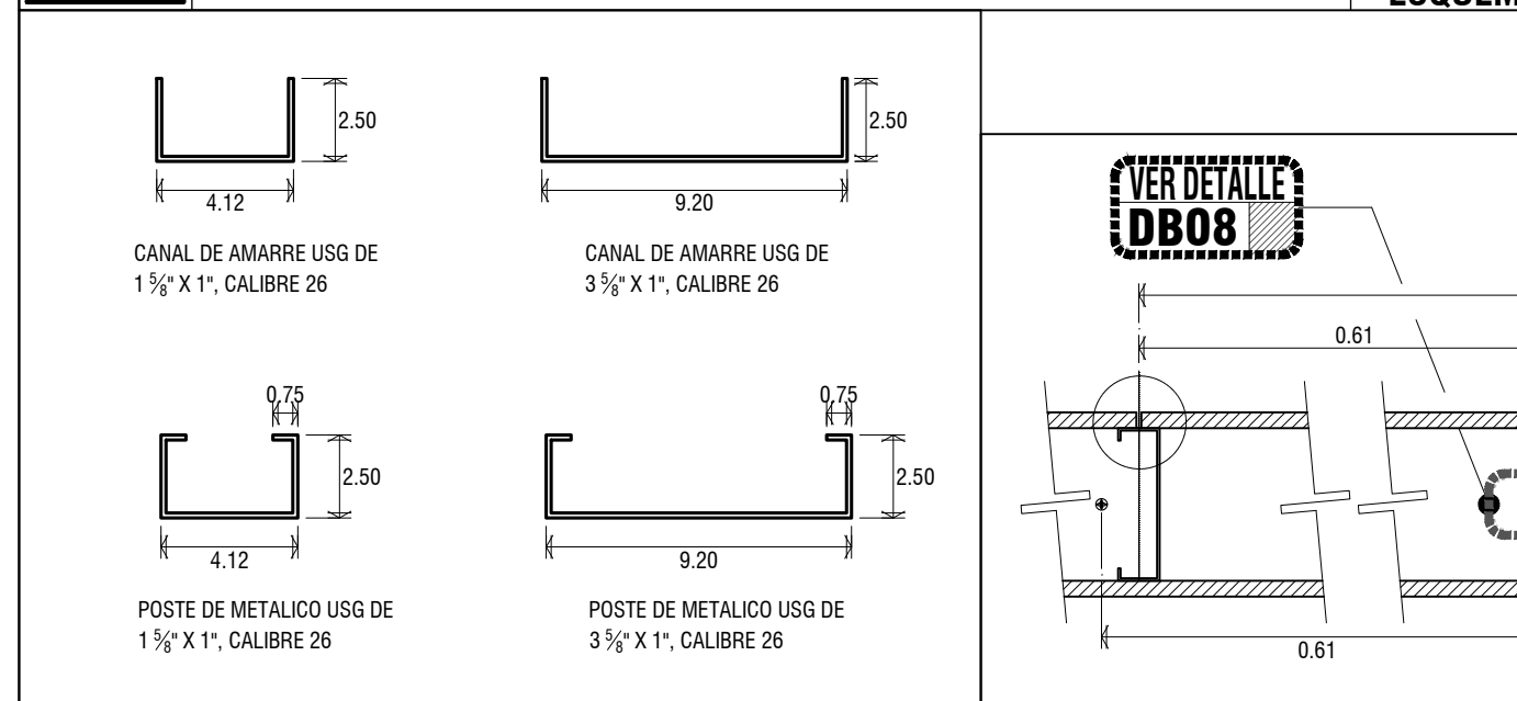
DB03 DETALLE DE PERFILES USG PARA TABLAROCA ESCHEMA
