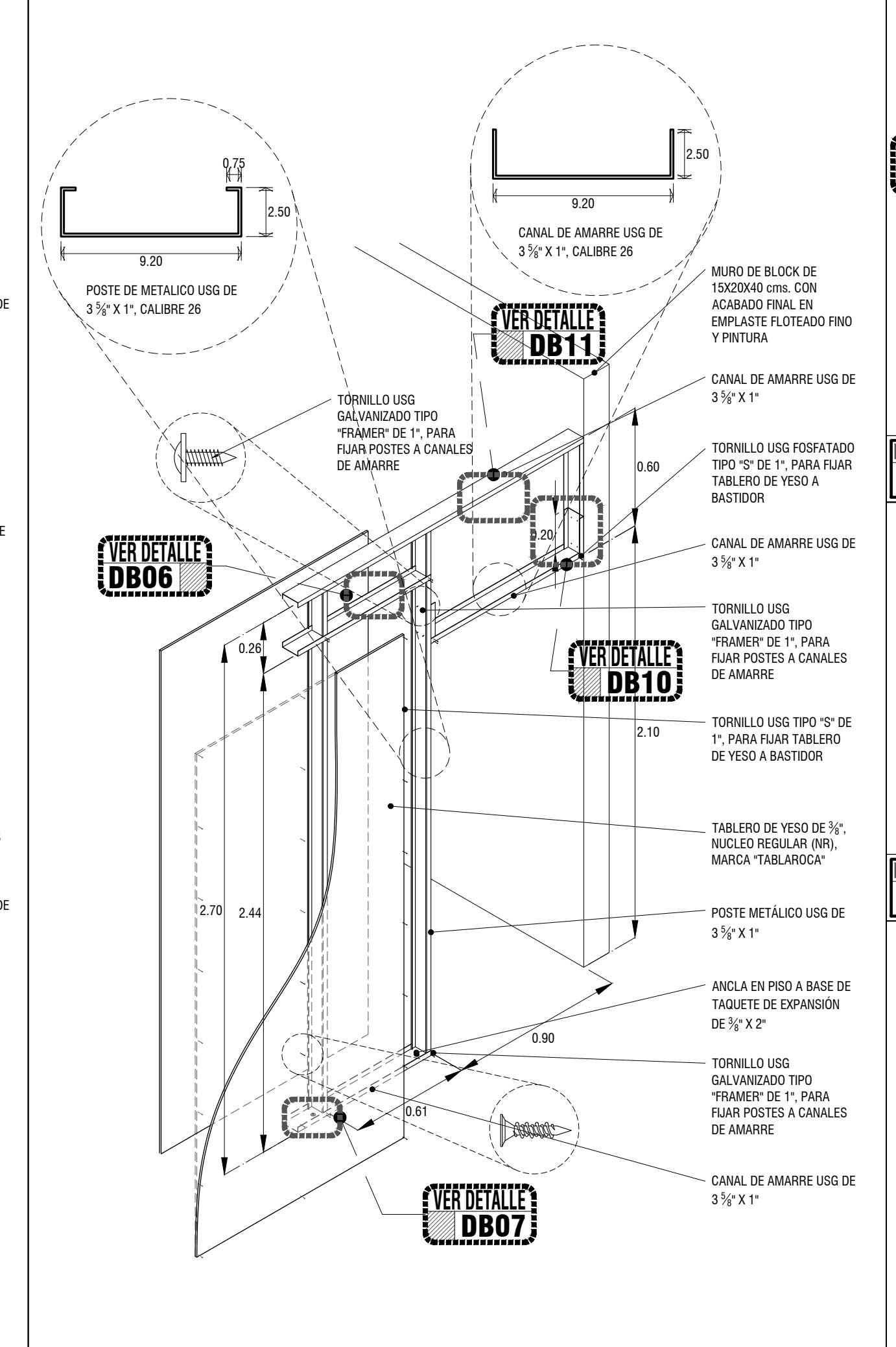
DB05 DETALLE DE ARMADO DE VANO EN MURO DE TABLAROCA ESC: 1:25
