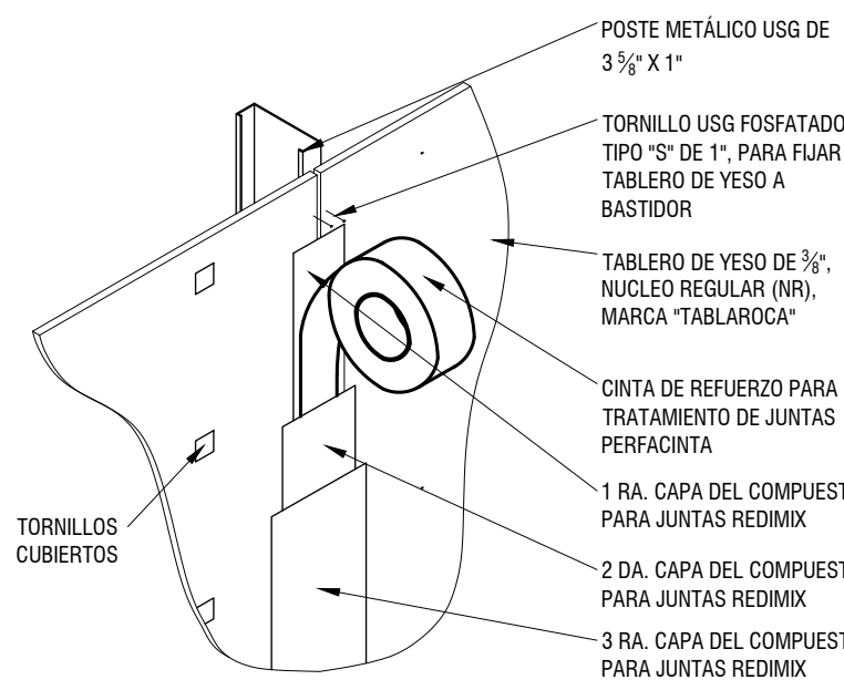
DB13 DETALLE DE TRATAMIENTO DE JUNTAS DE MURO DE TABLAROCA ESC: 1 : 5
