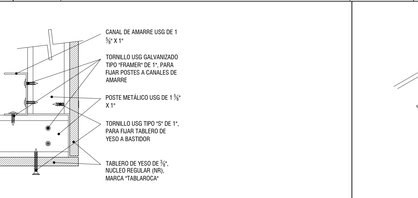
DB12 DETALLE DE AMARRE EN ESQUINA DE PERFILES DE MURO DE TABLAROCA ESCHEMA
