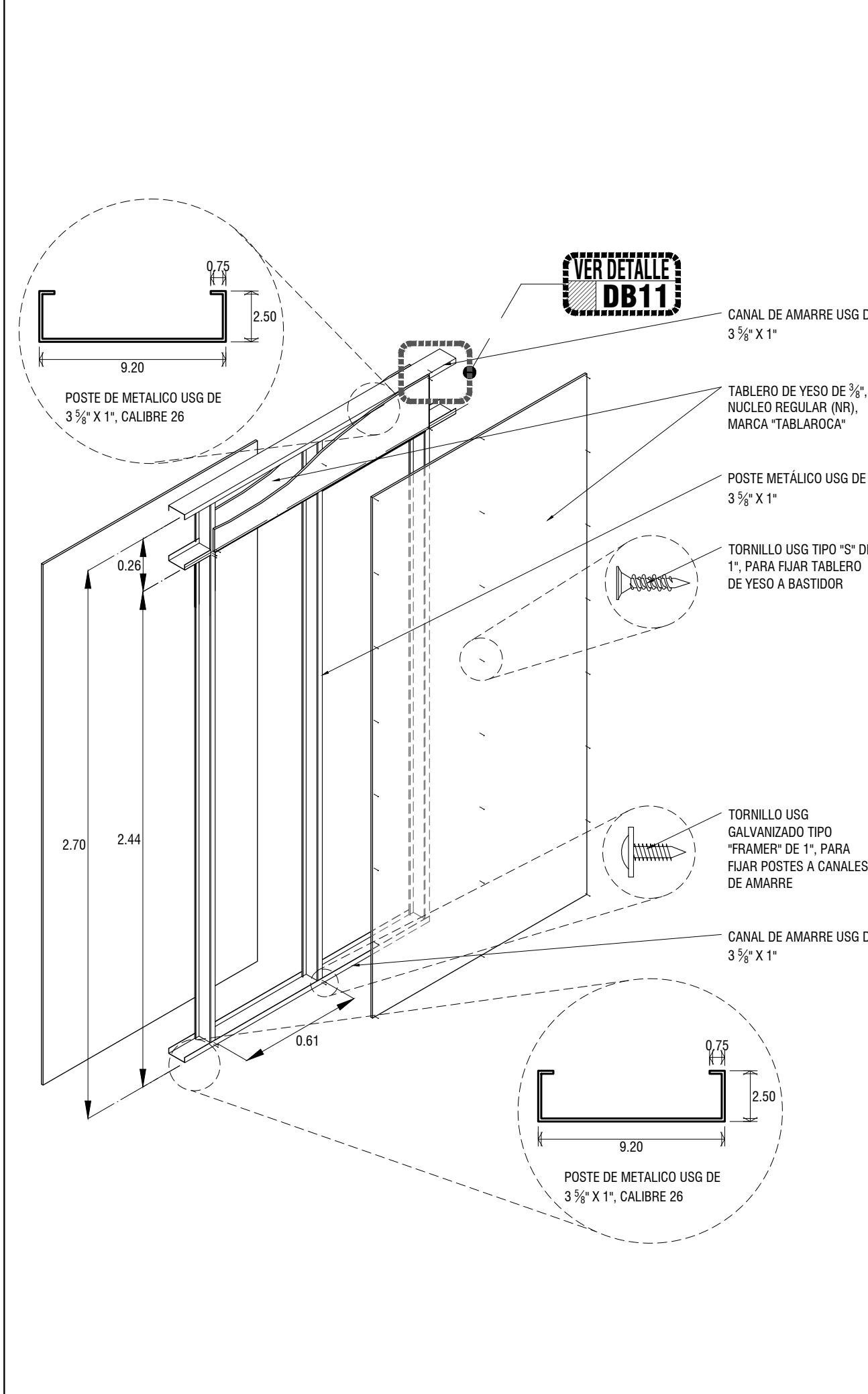
DB04 DETALLE DE ARMADO GENERAL DE MURO DE TABLAROCA ESC: 1:25
