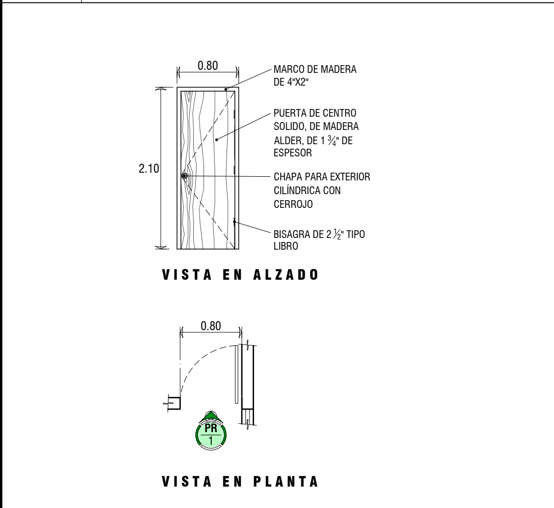
CR01 DETALLE DE PLANTA DE CARPINTERIA DE PUERTAS PLANTA BAJA ESC: 1:125
