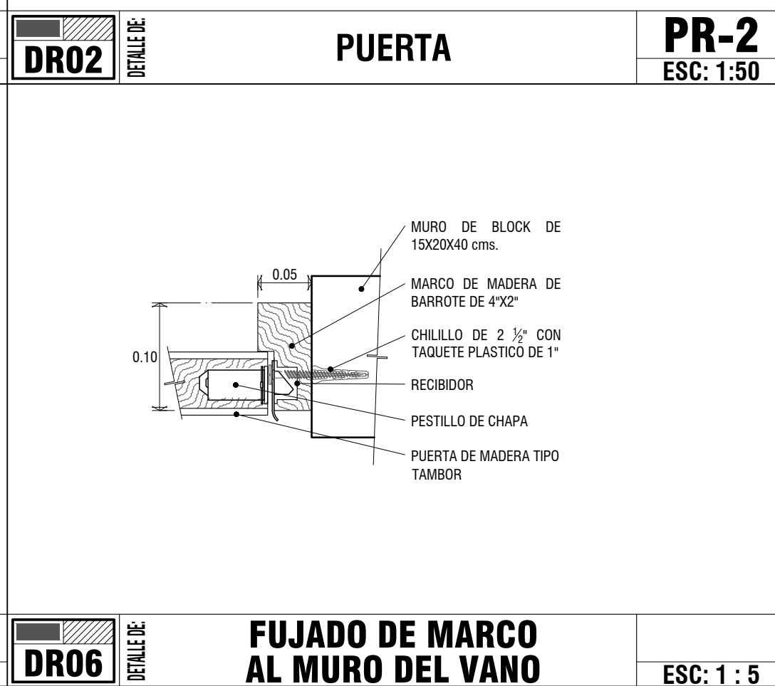
DR06 DETALLE DE FUJADO DE MARCO AL MURO DEL VANO ESC: 1 : 5
