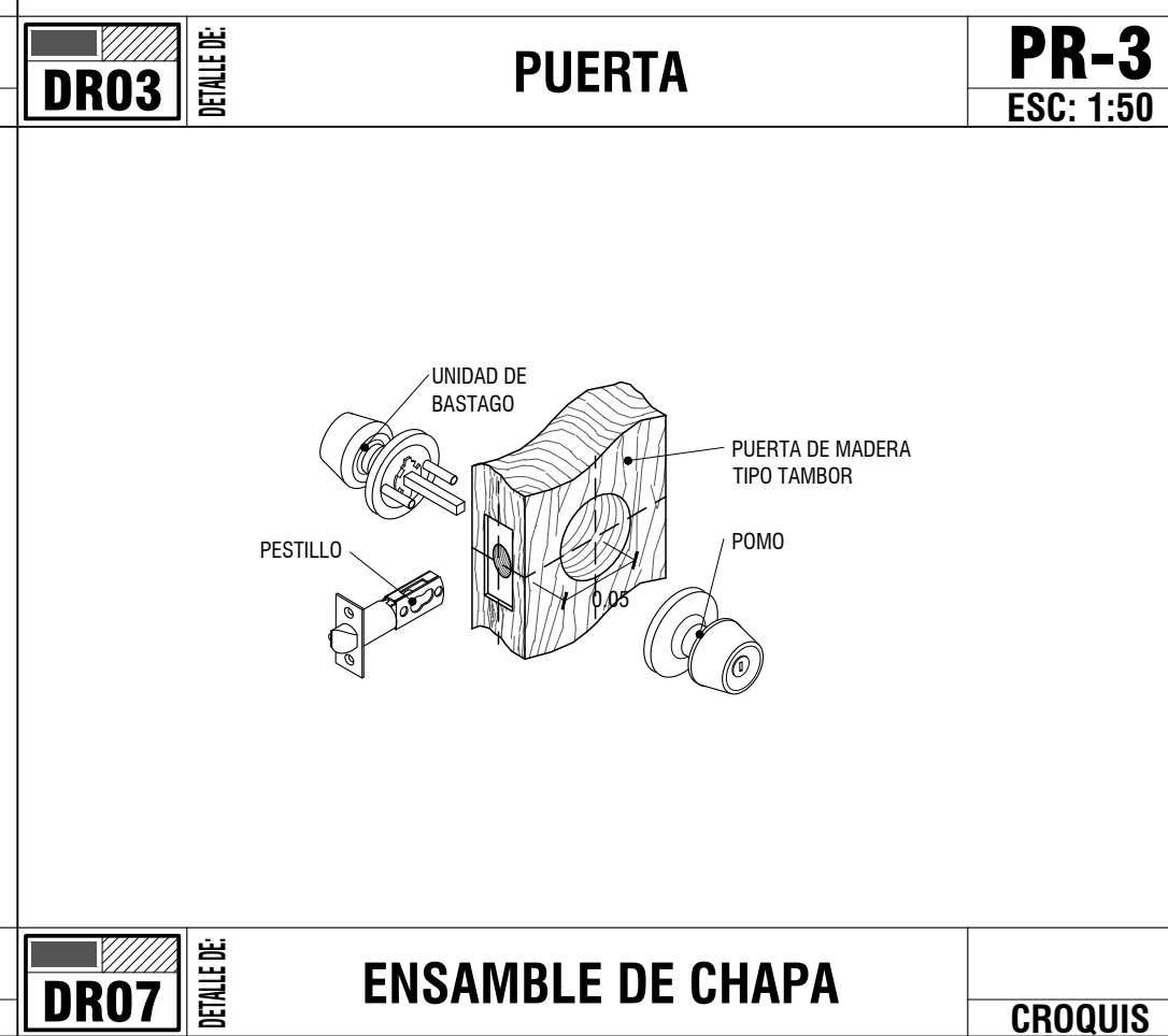
DR07 DETALLE DE ENSAMBLE DE CHAPA CROQUIS
