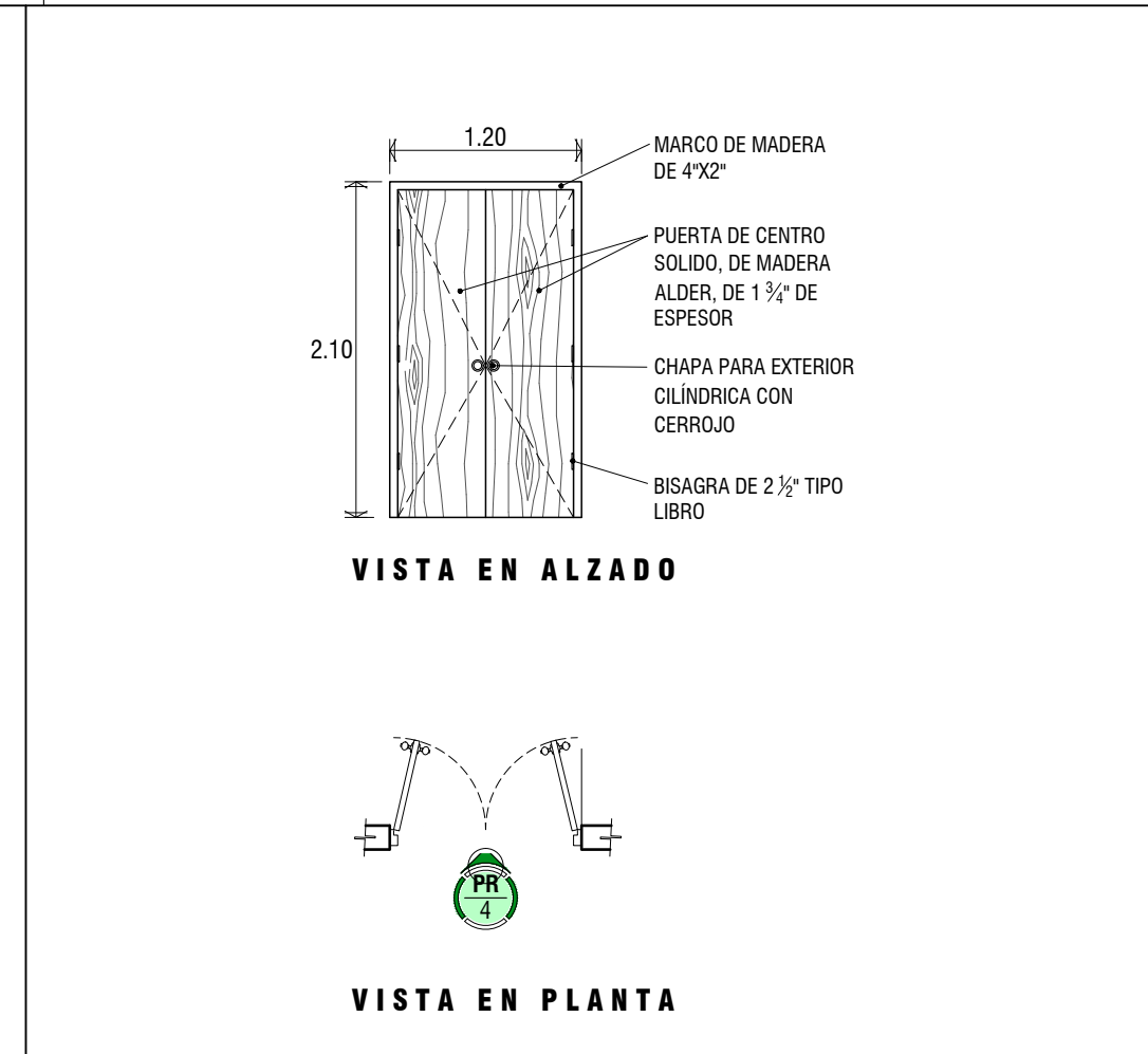
CA02 DETALLE DE PLANTA DE CANCELERIA DE PUERTAS PLANTA ALTA ESC: 1:125
