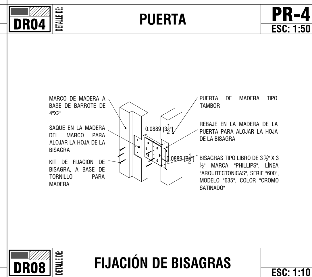
DR08 DETALLE DE FIJACION DE BISAGRAS ESC: 1:10
