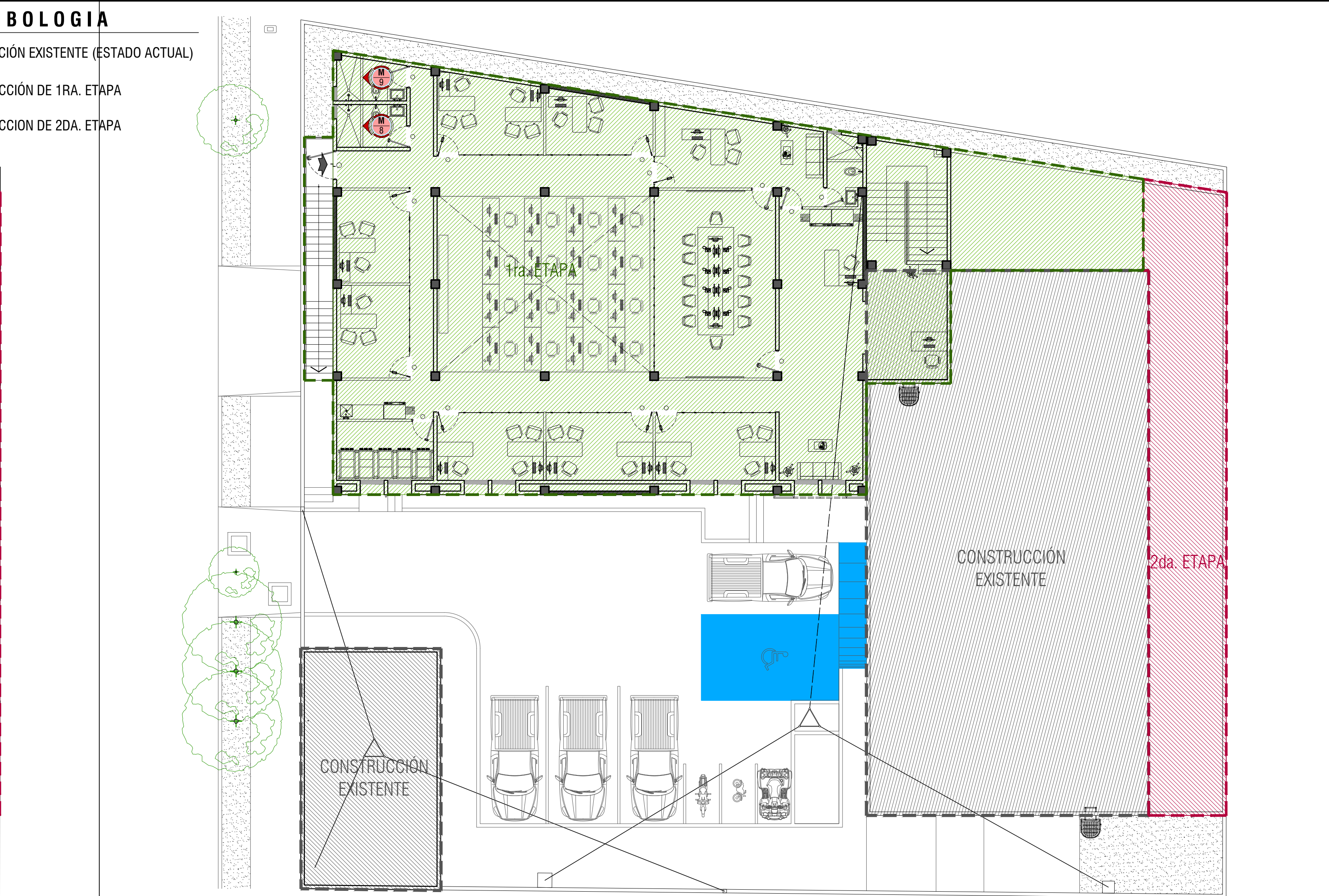
CA02 PLANTA DE CANCELERIA DE PUERTAS PLANTA ALTA ESC: 1:125
