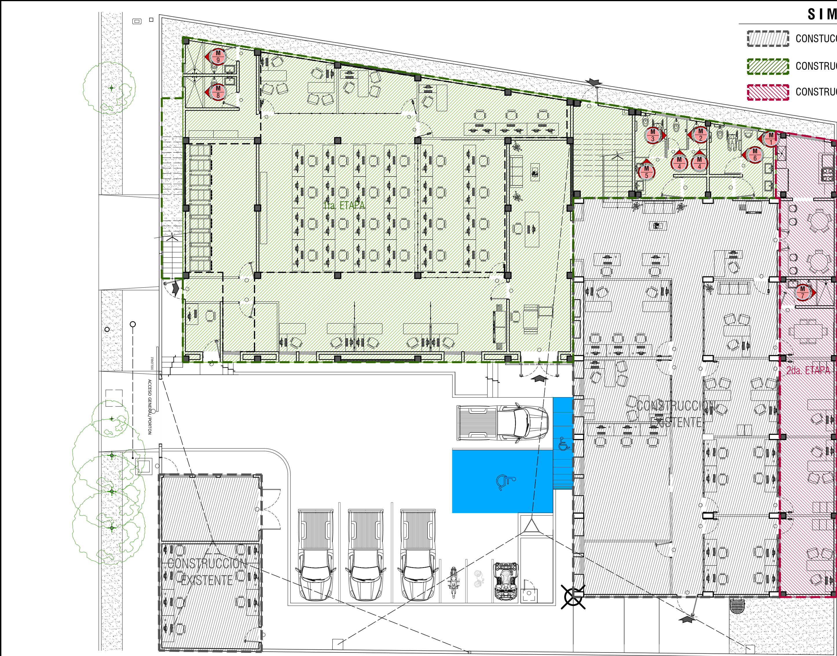
CA01 PLANTA DE CANCELERIA DE PUERTAS PLANTA BAJA ESC: 1:125
