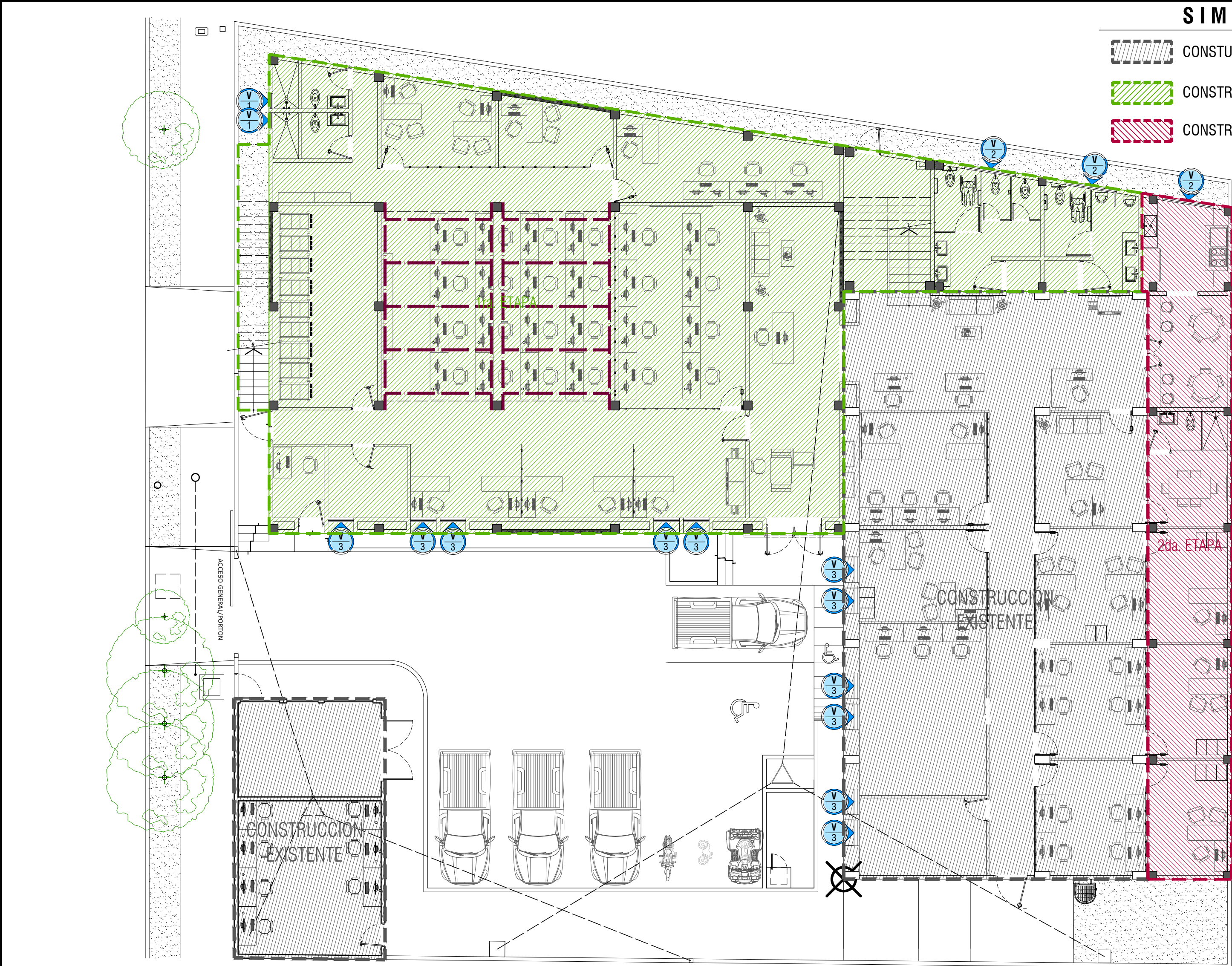
PLANTA DE CANCELERIA DE VENTANAS EXTERIORES PLANTA BAJA
