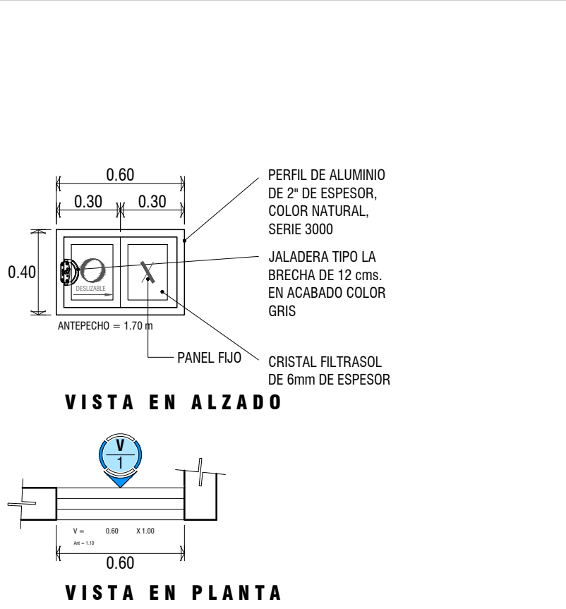
PLANTA DE CANCELERIA DE VENTANAS EXTERIORES PLANTA BAJA
