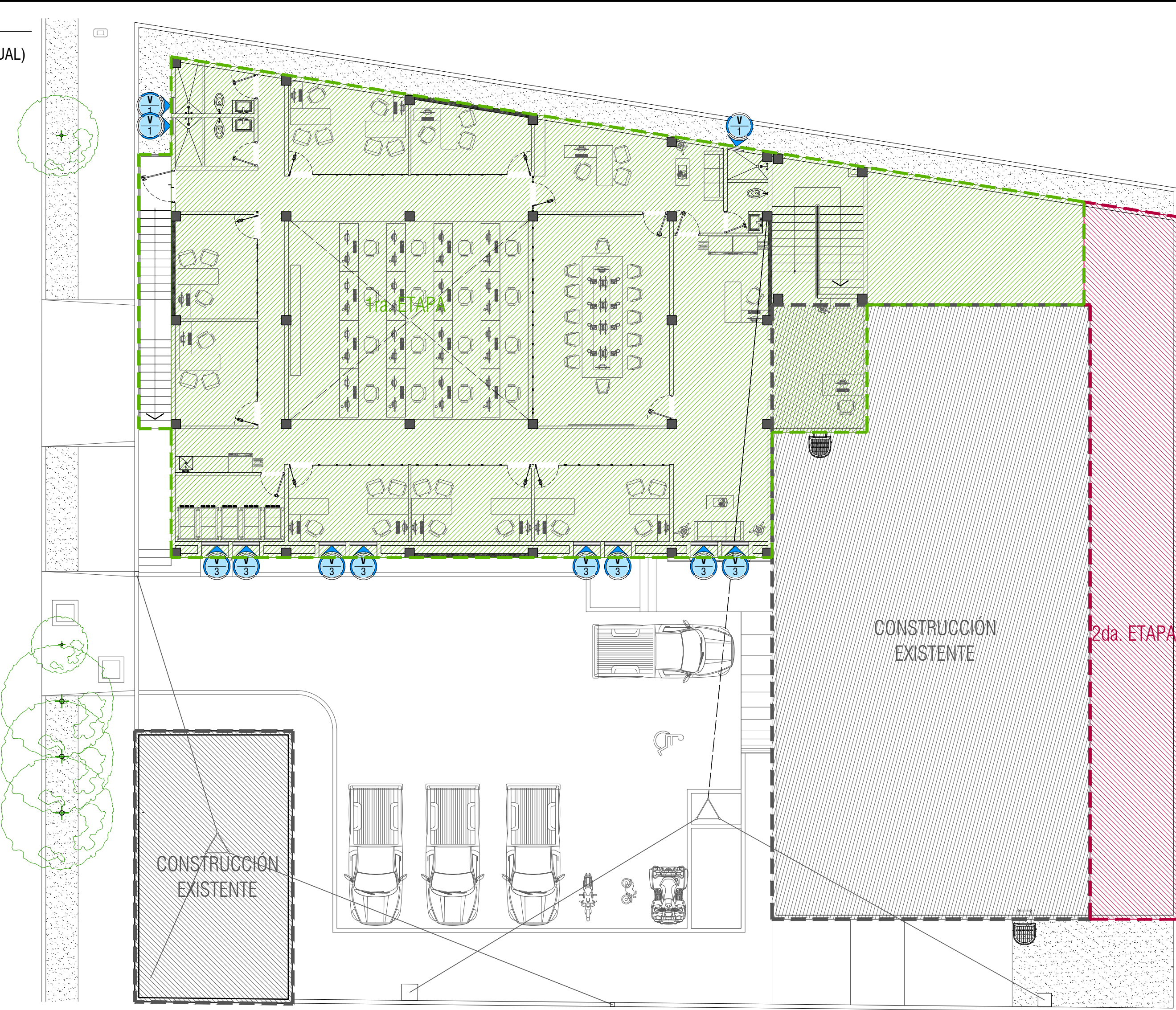
PLANTA DE CANCELERIA DE VENTANAS EXTERIORES PLANTA ALTA
