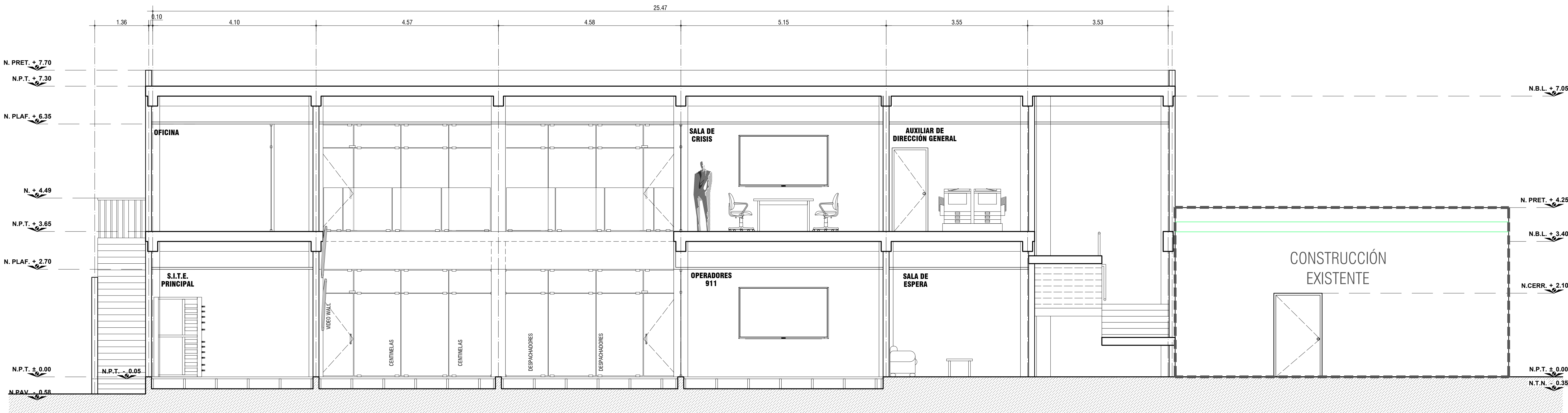
AQ05 CORTE LONGITUDINAL A - A' C4 LA PAZ ESCALA: 1:50 / ACOT: En mts.
