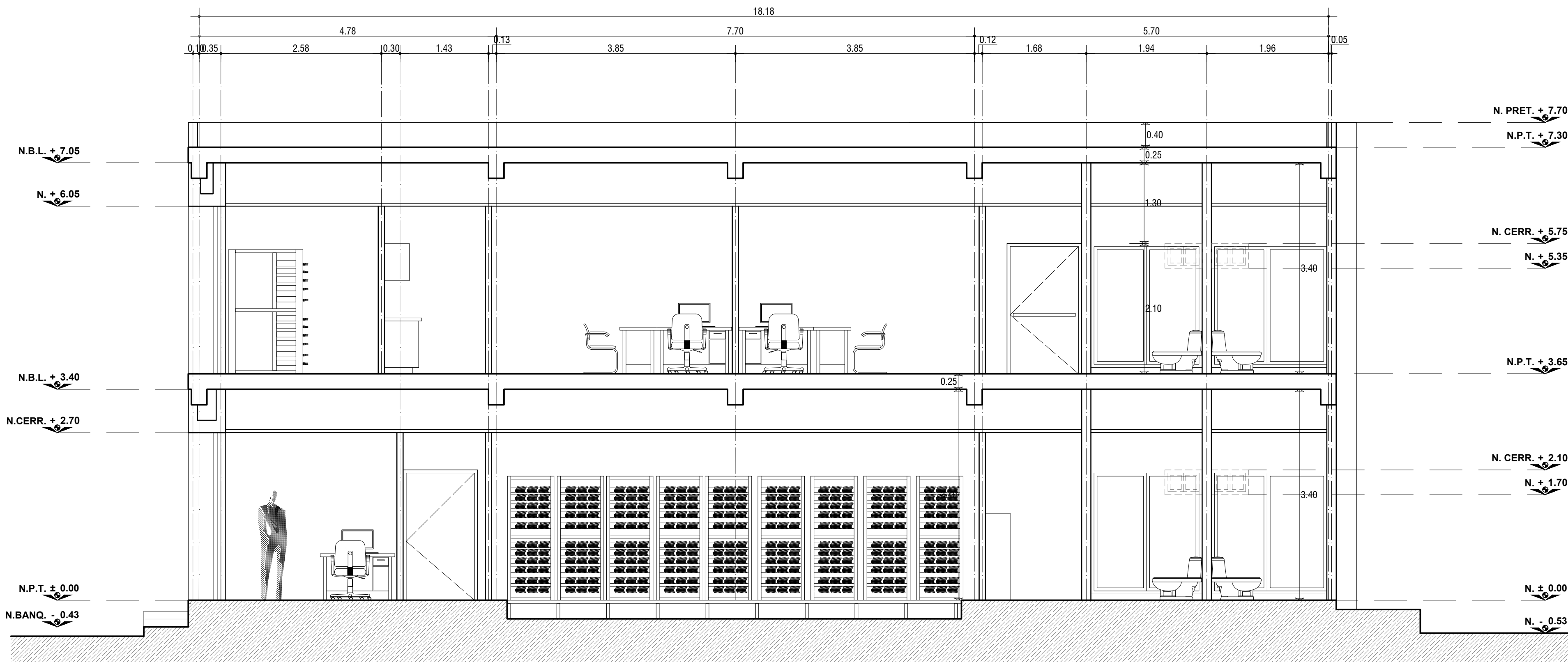
AQ06 CORTE TRANSVERSAL B - B' C4 LA PAZ ESCALA: 1:50 / ACOT: En mts.
