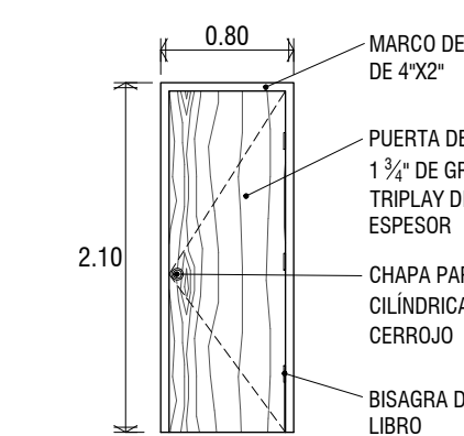
VISTA EN ALZADO
