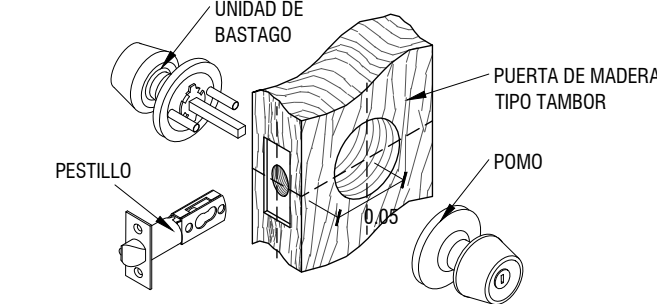
DR06 DETALLE DE ENSAMBLE DE CHAPA CARPINTERIA Escala: Croquis
