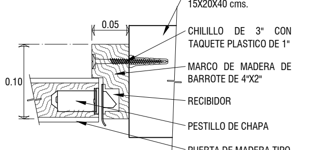
DR07 DETALLE DE MARCO DE PUERTA CARPINTERIA Escala: Croquis
