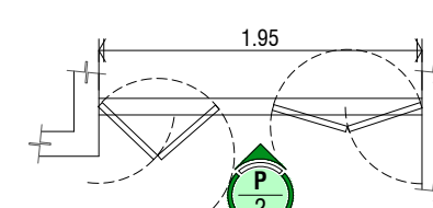
DR04 DETALLE DE PUERTA P-4 PUERTAS ESCALA: 1:50
