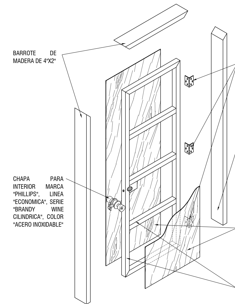
DR05 ESQUEMA DE ENSAMBLE DE PUERTA CARPINTERIA Escala: Croquis
