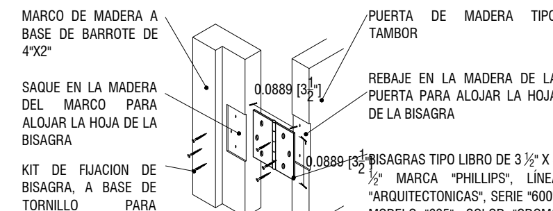
DR08 DETALLE DE FIJACION DE BISAGRAS CARPINTERIA Escala: 1:10
