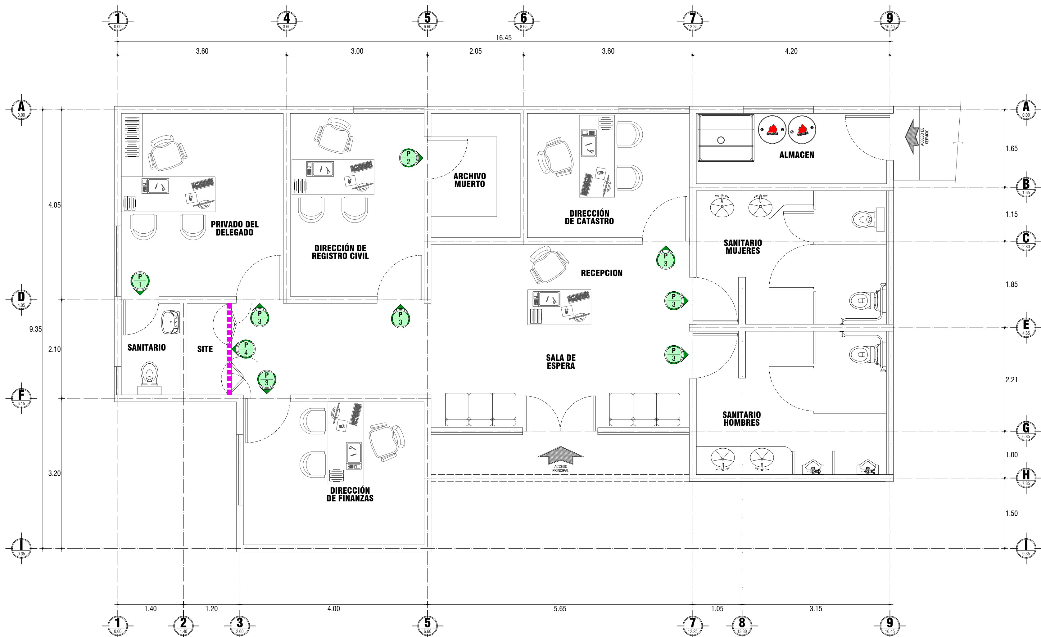
CR01 PLANTA DE CARPINTERIA PUERTAS DELEGACION MPAL. PTO. ADOLFO L.M. ESCALA: 1:50 / ACOT: En mts.
