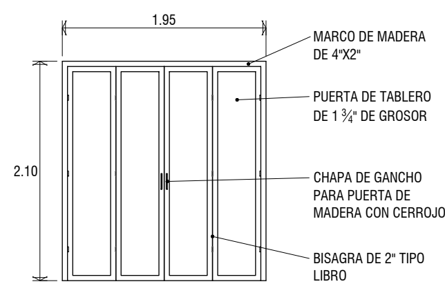
VISTA EN ALZADO
