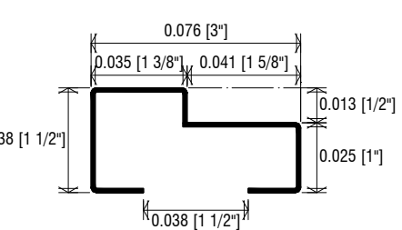
PERFIL M-300 DETALLE Escala: Croquis
