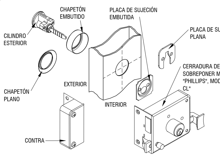
DETALLE DE ENSAMBLE DE CHAPA CARPINTERIA Escala: Croquis
