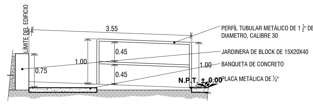
BARANDAL BH1 RAMPA PARA PERSONAS CON DISCAPACIDAD DETALLE ESCALA: 1:50 / ACOT: En mts.
