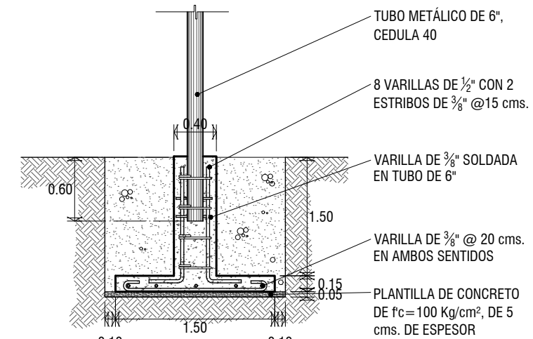
ZAPATA AISLADA ASTA BANDERA DETALLE ESCALA: 1:50 / ACOT: En mts.
