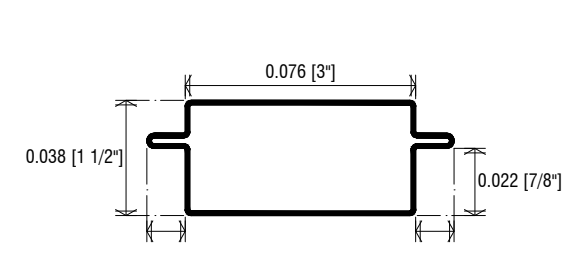
PERFIL K-300 DETALLE Escala: Croquis
