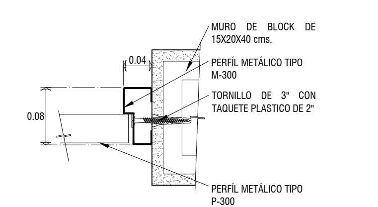
DETALLE DE MARCO DE PUERTA CARPINTERIA Escala: Croquis
