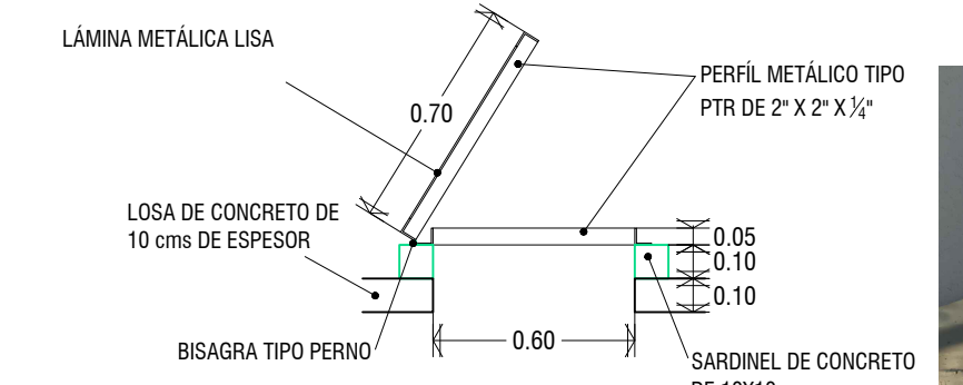
VISTA EN SECCIÓN
