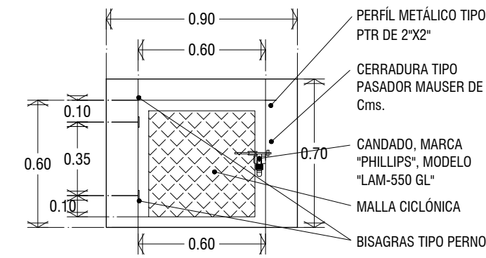
VISTA EN ALZADO FRONTAL
