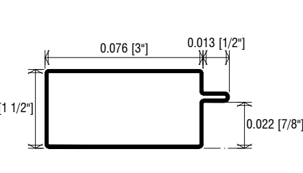
PERFIL P-300 DETALLE Escala: Croquis
