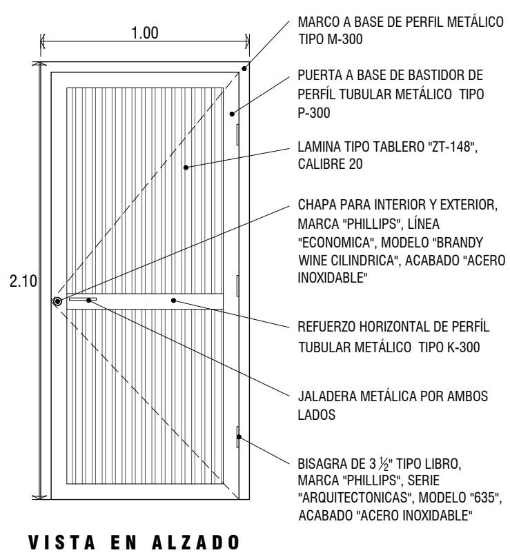
VISTA EN ALZADO
