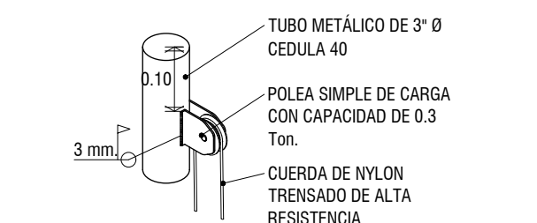
FIJACIÓN DE POLEA DETALLE ESCALA: 1:10 / ACOT: En mts.
