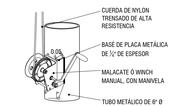
MALACATE O WINCH MANUAL DETALLE ESCALA: 1:10 / ACOT: En mts.
