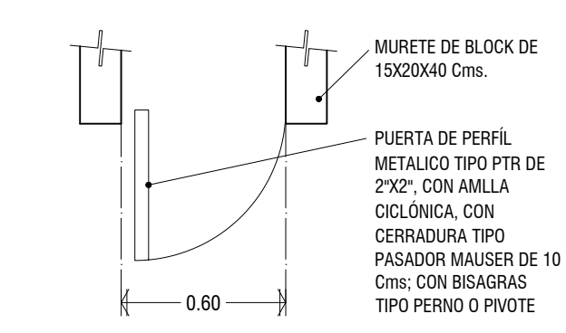
PUERTA DE BOMBA DETALLE ESCALA: 1:25 / ACOT: En mts.
