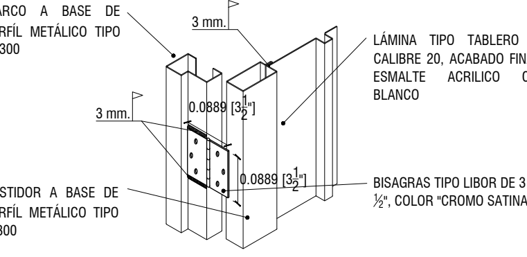
DETALLE DE FIJACION DE BISAGRAS CARPINTERIA Escala: 1:10
