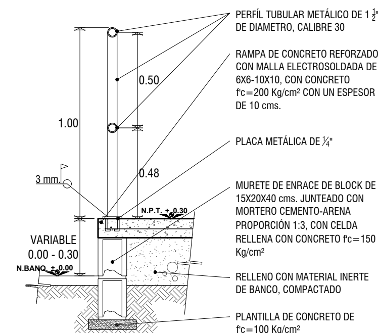
BARANDAL PARA RAMPA DETALLE ESCALA: 1:20 / ACOT: En mts.
