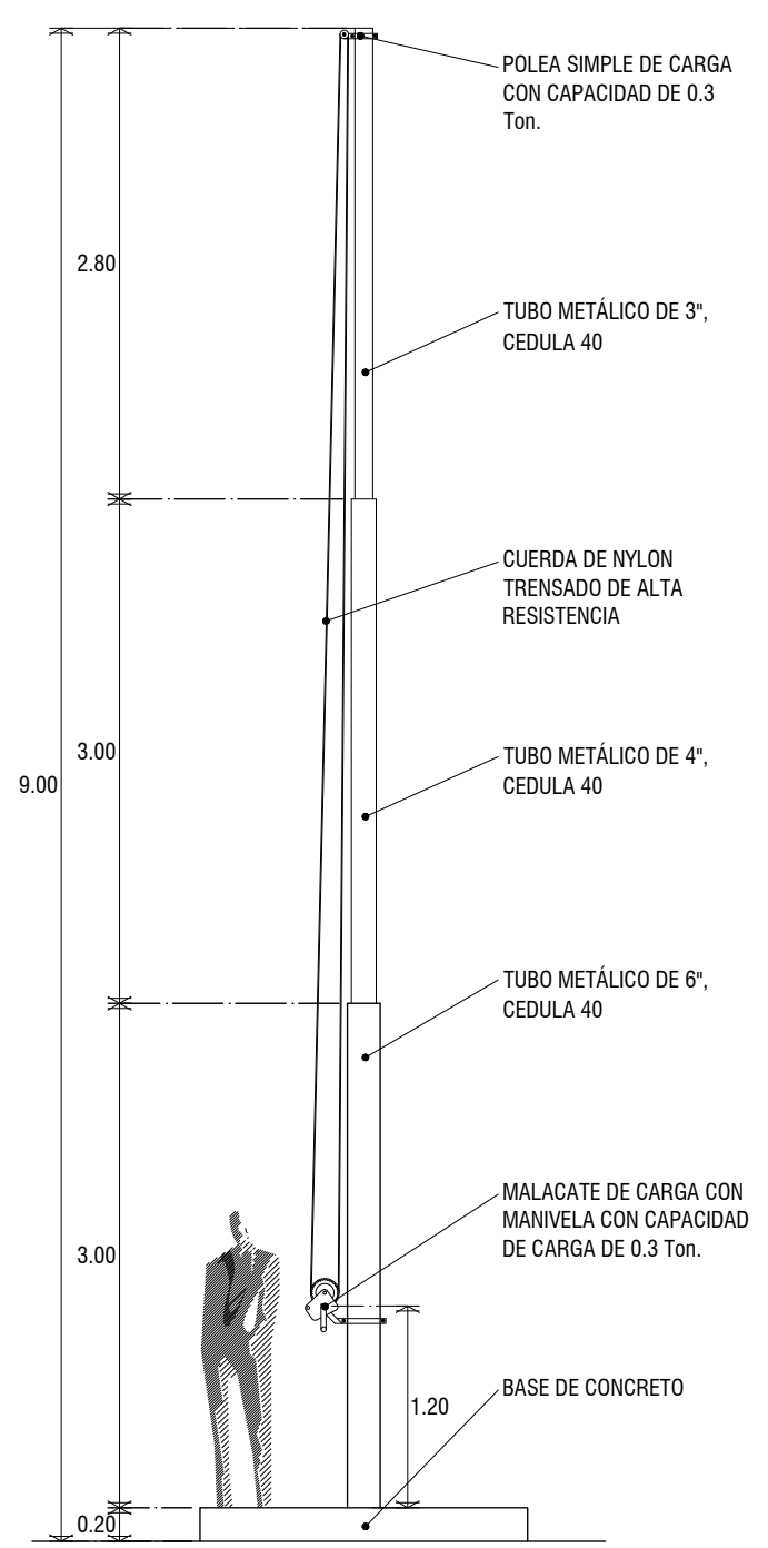
ASTA BANDERA DETALLE ESCALA: 1:50 / ACOT: En mts.
