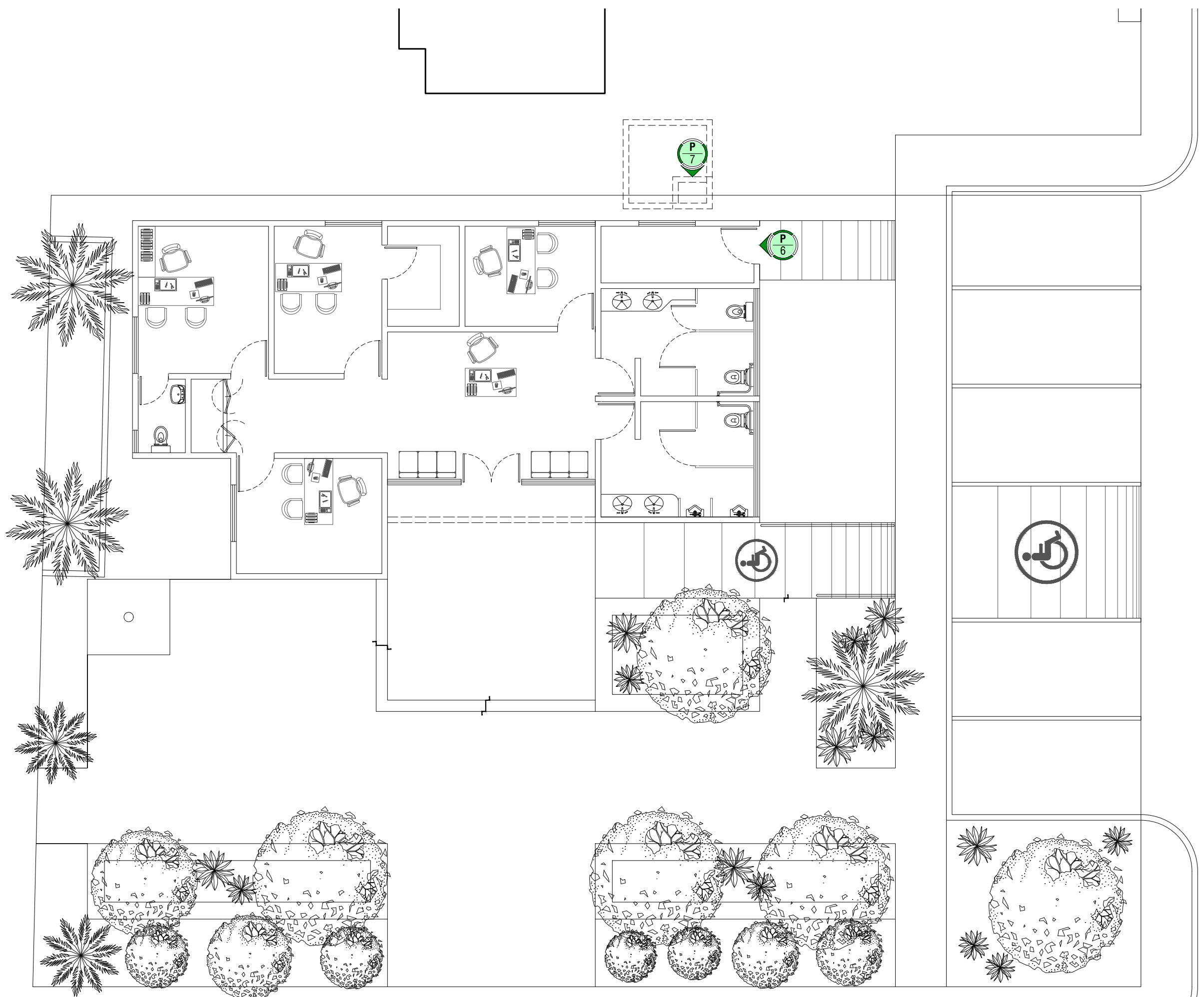
PLANTA DE HERRERIA DELEGACION MPAL. PTO. ADOLFO L.M. ESCALA: 1:100 / ACOT: En mts.
