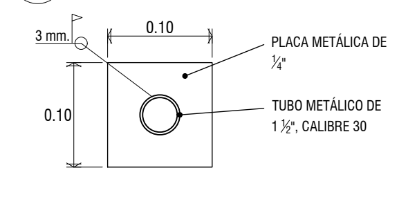
PLACA PARA BARANDAL DETALLE ESCALA: 1:25 / ACOT: En mts.
