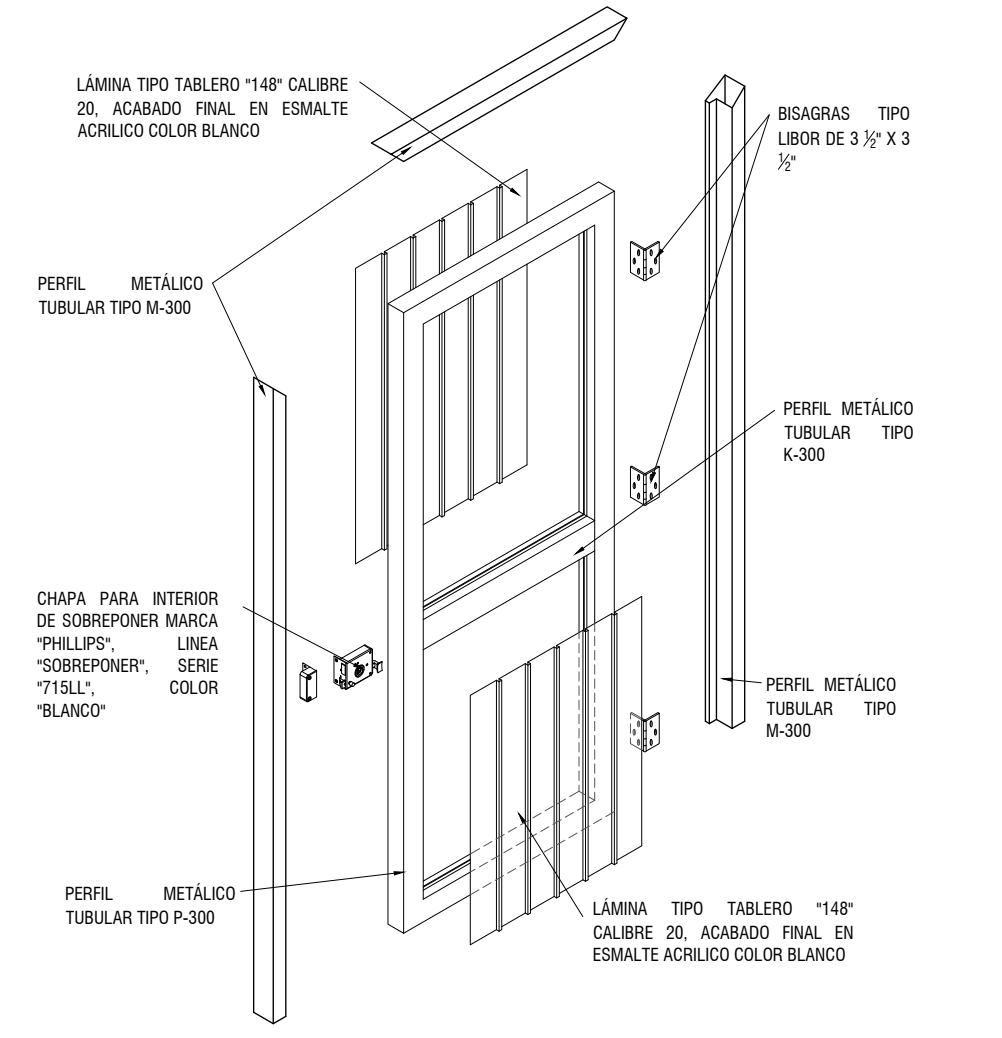
ESQUEMA DE ENSAMBLE DE PUERTA HERRERIA Escala: Croquis
