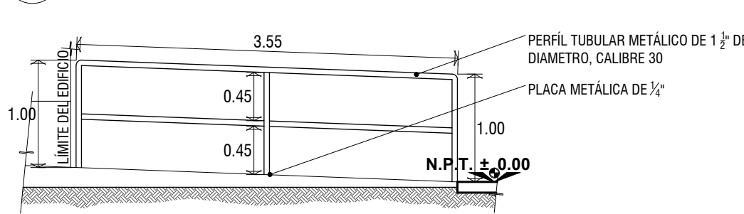
BARANDAL BH2 RAMPA PARA PERSONAS CON DISCAPACIDAD DETALLE ESCALA: 1:50 / ACOT: En mts.
