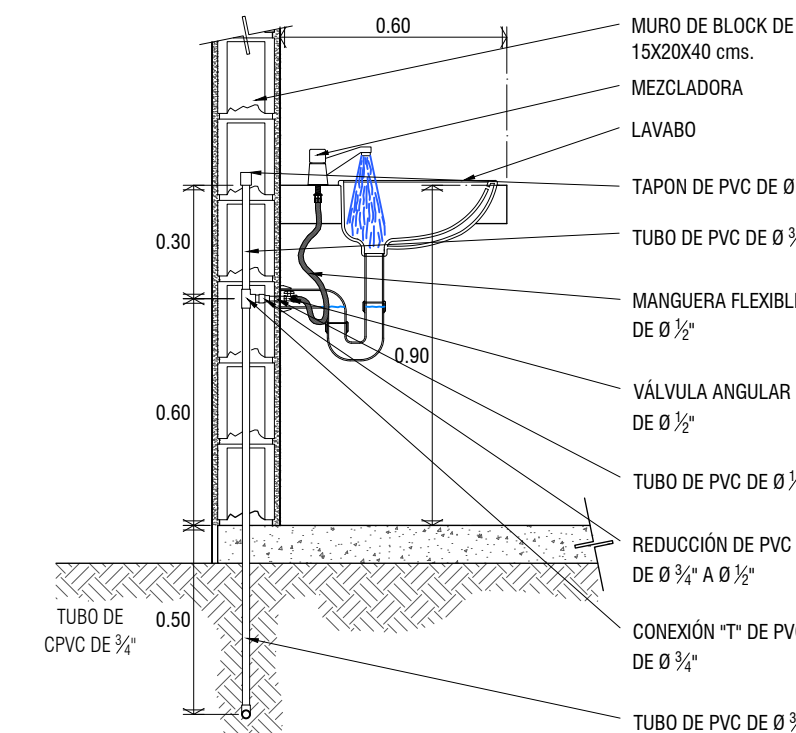
DETALLE DE CONEXION HIDRÁULICA LAVABO
