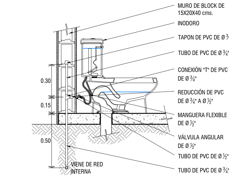
DETALLE DE CONEXIÓN HIDRÁULICA INODORO
