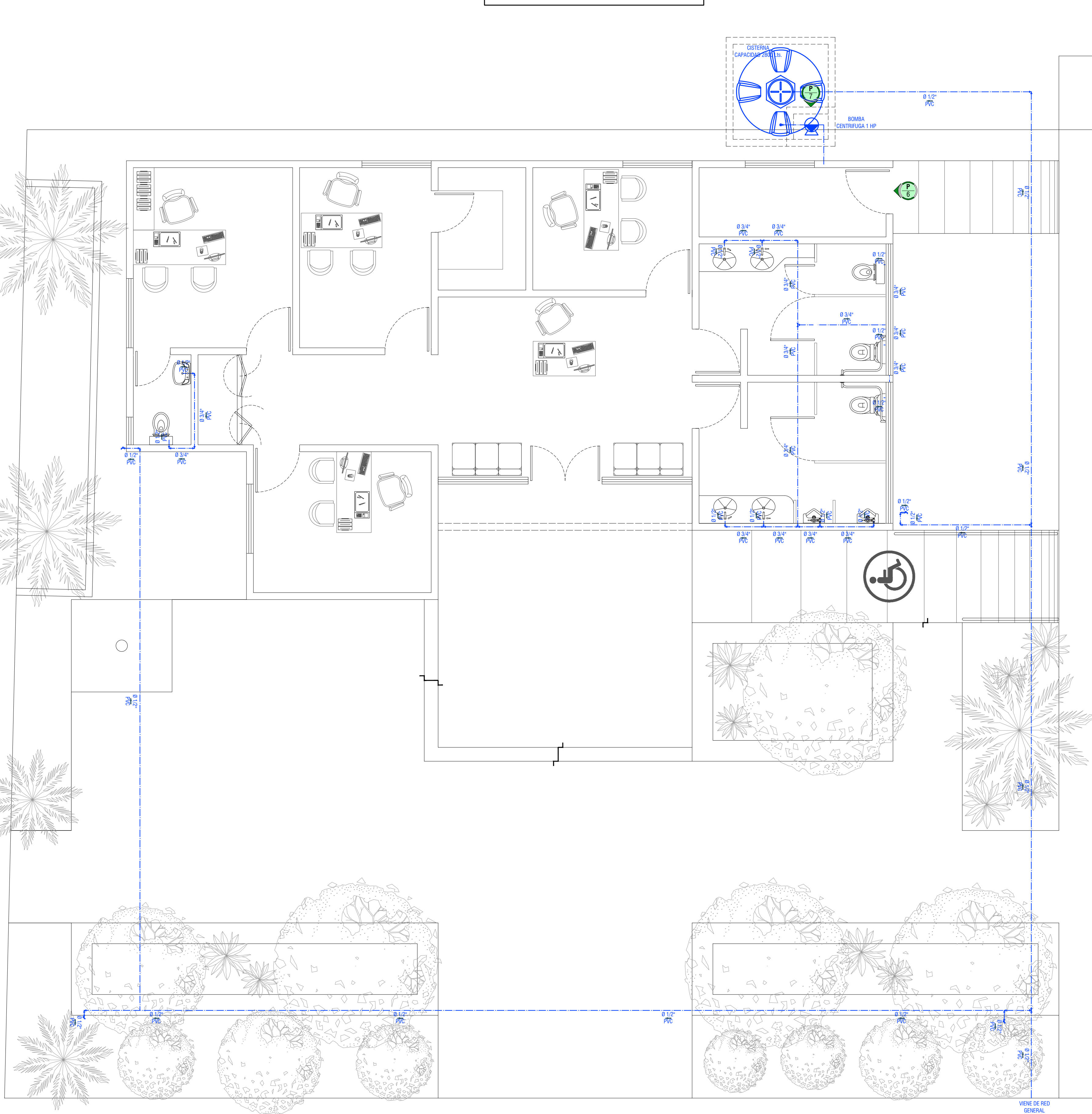
PLANTA DE INSTALACIÓN HIDRAULICA DELEGACION MPAL. PTO. ADOLFO L.M. ESCALA: 1:50 / ACOT: En mts.
