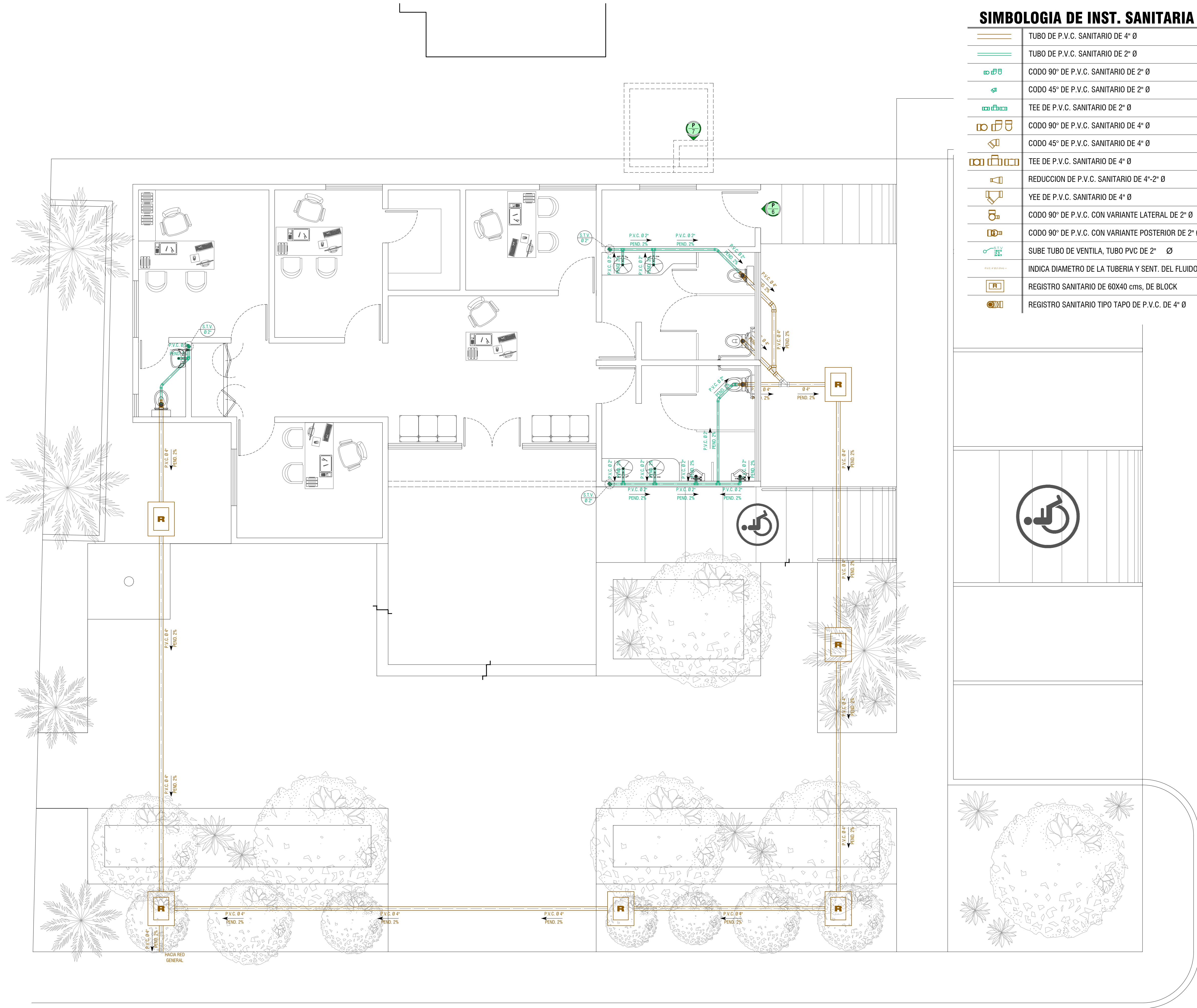
IS01 PLANTA DE INSTALACIÓN SANITARIA DELEGACION MPAL. PTO. ADOLFO L.M. ESCALA: 1:50 / ACOT: En mts.
